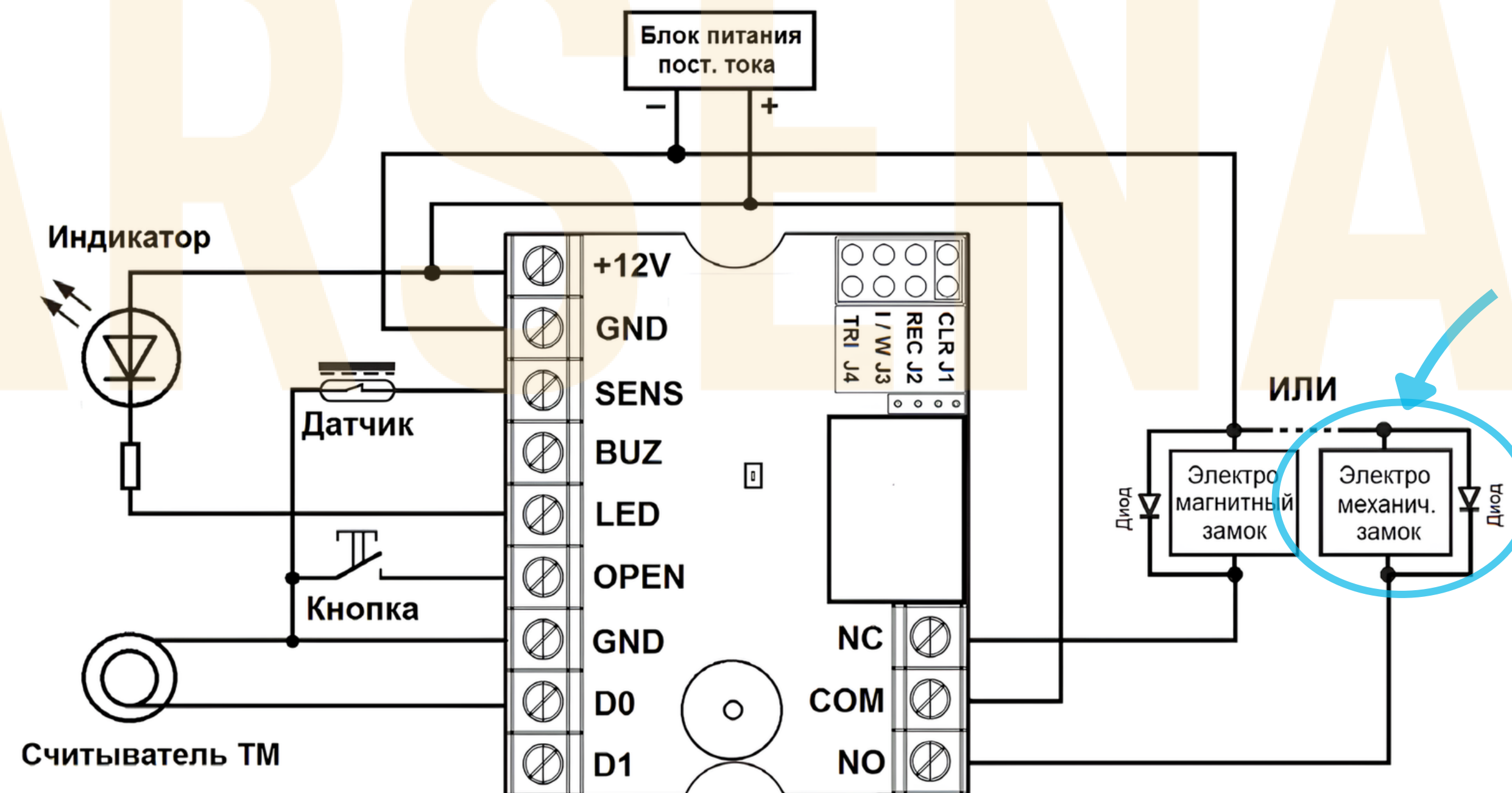
ПРИМЕР ПОДКЛЮЧЕНИЯ К КОНТРОЛЛЕРУ
