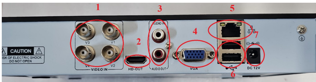
1.1. Подключаем видеорегистратор к сети и питанию.
