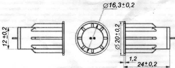
Рис. 1 Габаритные и установочные размеры.
