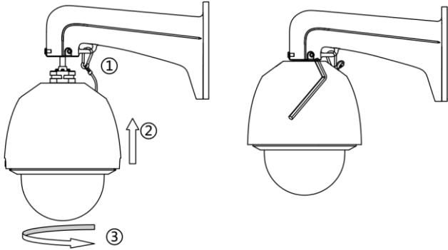
Рисунок 1-9 Установка скоростной поворотной камеры
