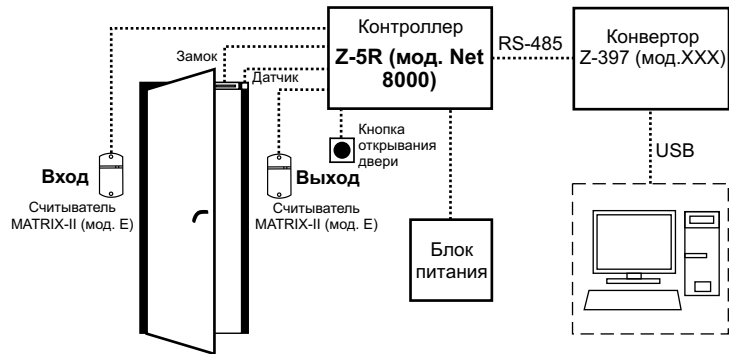
Рис.1 Схема СКУД с контроллером Z-5R (mod. Net 8000)
