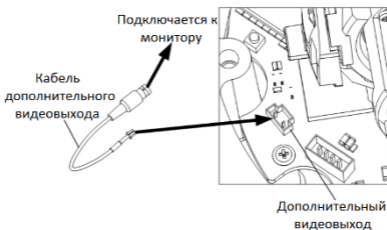
Рисунок 2-8 Подключение камеры к монитору
